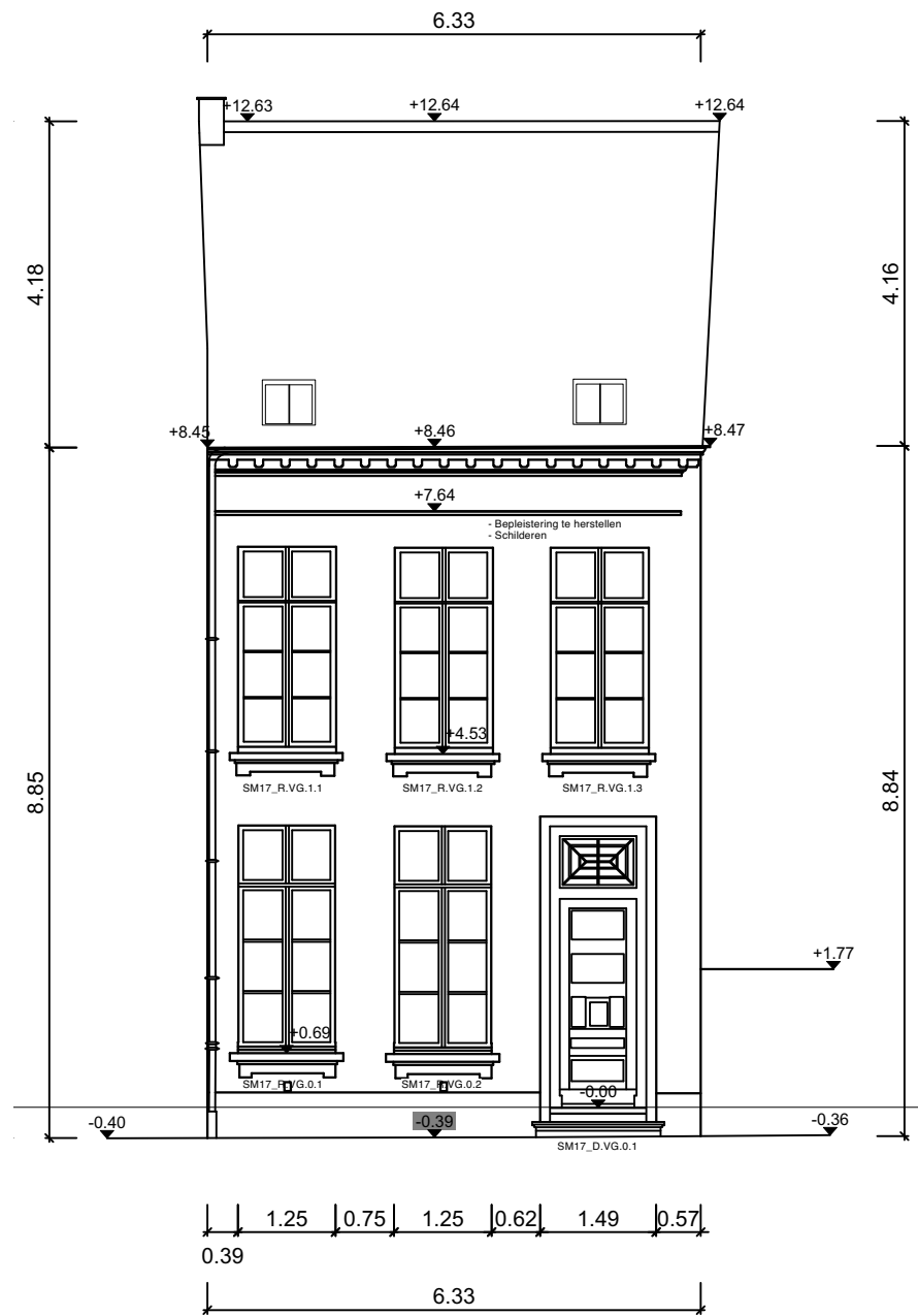
VOORGEVEL
