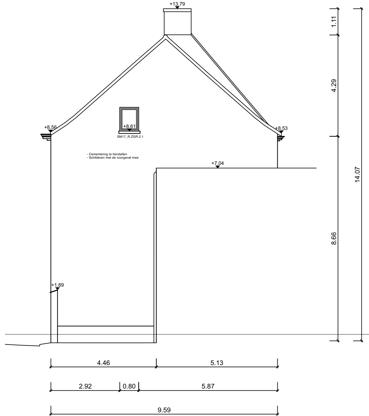
ZIJGEVEL RECHTS
