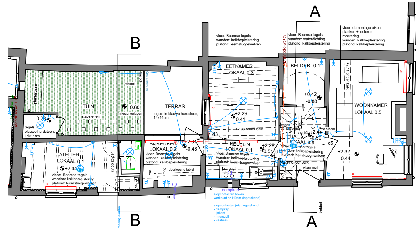
GELIJKVLOERS
