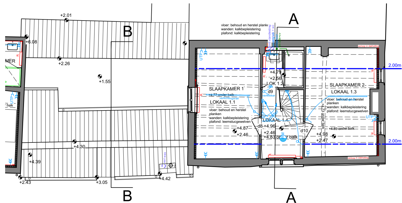
EERSTE VERDIEPING
