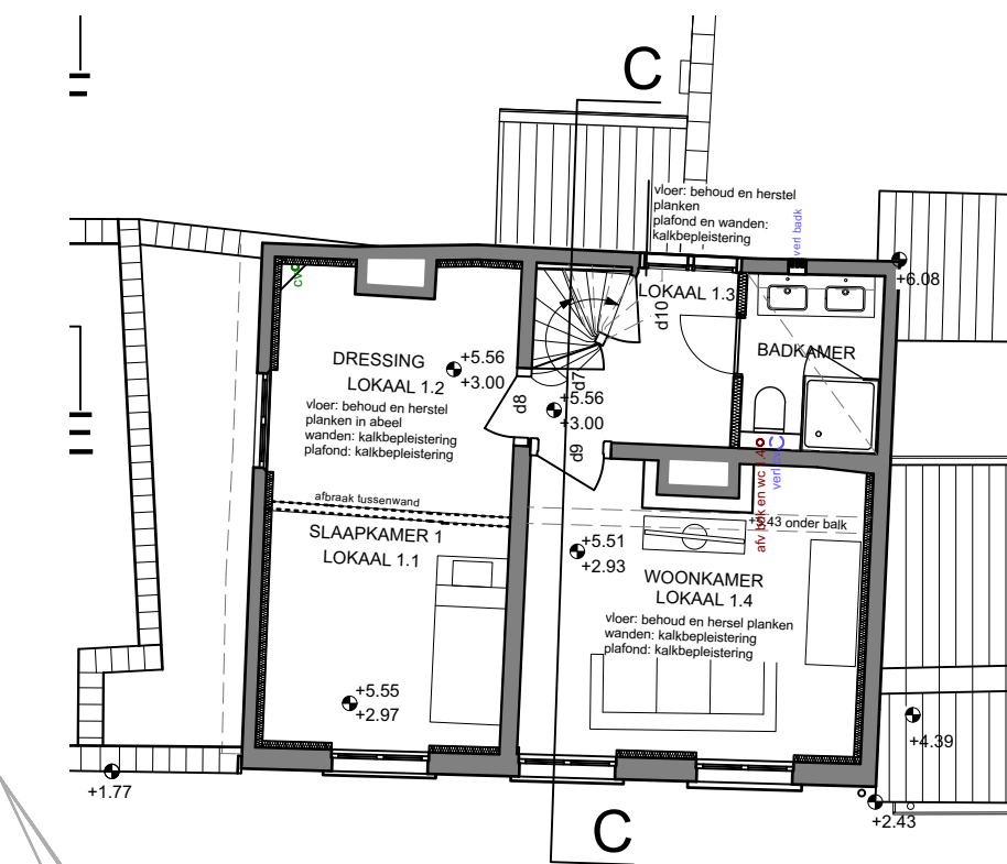
EERSTE VERDIEPING
