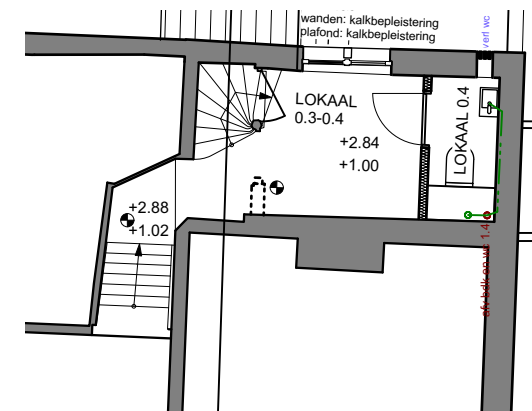
TUSSENVERDIEP
