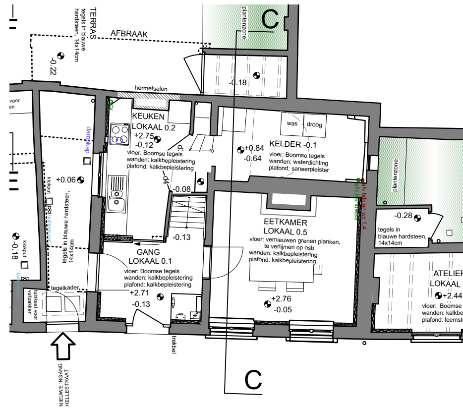
GELIJKVLOERS
